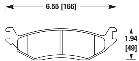
DODGE VAN (REAR)
