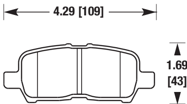
PONTIAC GRAND PRIX (REAR)
