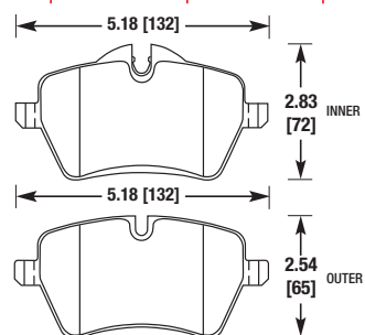
MINI COOPER (REAR)
