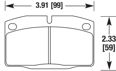
CARBONE LORRAINE 4012
