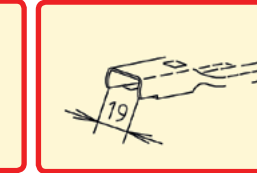
Рычаг под установку коннектора типа E
