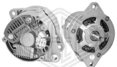
A125 - 14V - 55A
