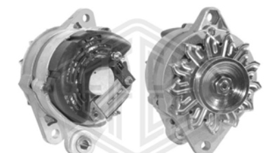
A125 - 14V - 55A - pulley Trapez. 1
