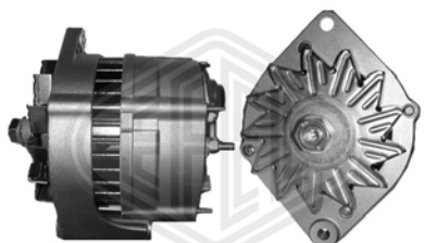
N1 - 28V - 80A - (fan wheel)
