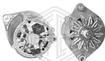
N1 - 28V - 80A - pulley Trapez. 1
