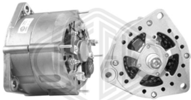
N1 - 28V - 80A
