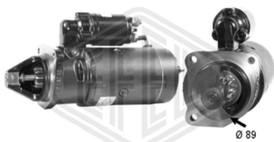
JF - 24V - 4kW - z 10
