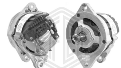
A125 - 28V - 30A
