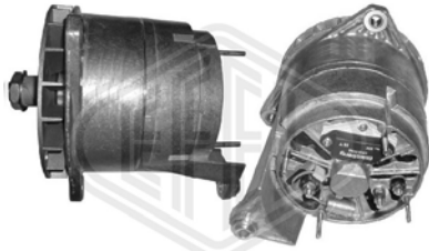
T1 - 28V - 140A - (Fan wheel)
