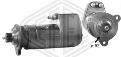
KB - 24V - 6.6kW - z 11
