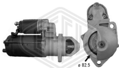
JF - 24V - 4kW - z 11
