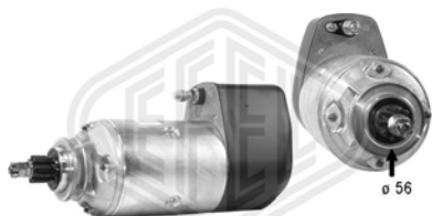
BNG - 24V - 4kW - z 9
