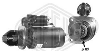
JF - 24V - 4kW - z 9
