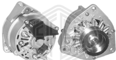
NL1 - 28V - 80A - pulley PolyV-9
