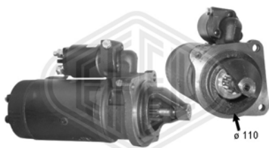
JF - 24V - 4kW - z 9
