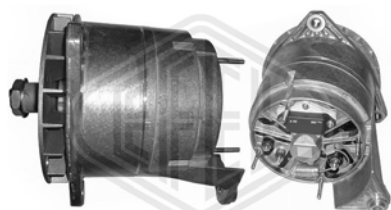
T1 - 28V - 140A - (Fan wheel)
