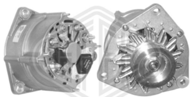
NL1 - 28V - 80A - pulley PolyV-8
