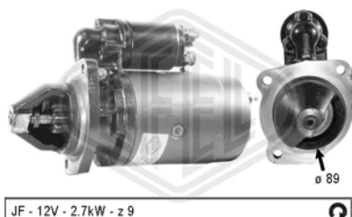
JF - 12V - 2.7kW - z 9
