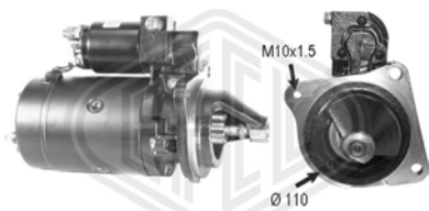
JF - 12V - 2.4kW - z 9
