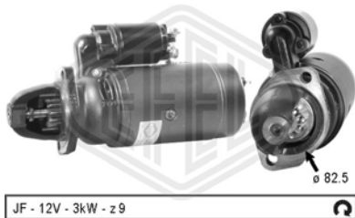
JF - 12V - 3kW - z 9
