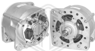
N1 - 28V - 65A
