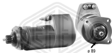
KB - 24V - 5.4kW - z 11
