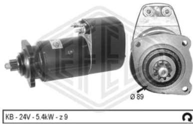
KB - 24V - 5.4kW - z 9
