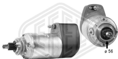
BNG - 12V - 3kW - z 9
