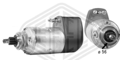
BNG - 24V - 4kW - z 11
