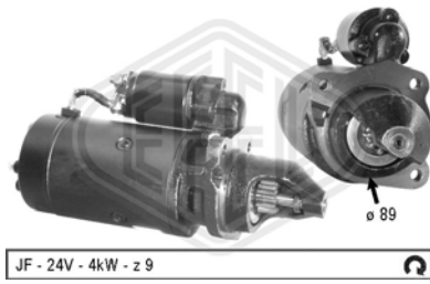
JF - 24V - 4kW - z 9
