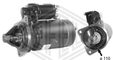
JF - 24V - 4kW - z 9
