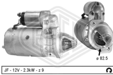
JF - 12V - 2.3kW - z 9
