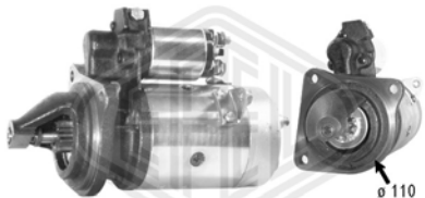
JF - 12V - 2kW - z 9
