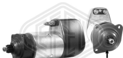
KB - 24V - 5.4kW - z 9
