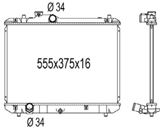
TYC 735-1003
