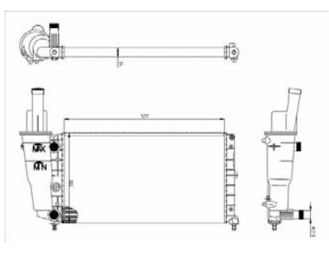
TYC 709-0007
