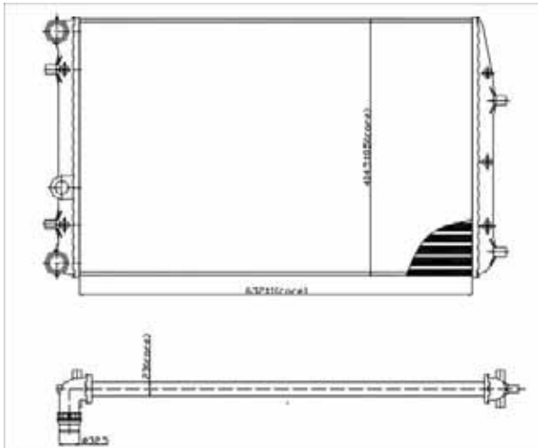
TYC 737-0041
