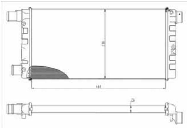
TYC 709-0008
