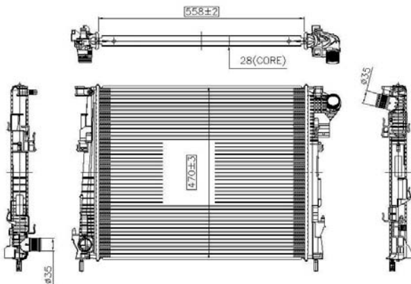
TYC 725-0032
