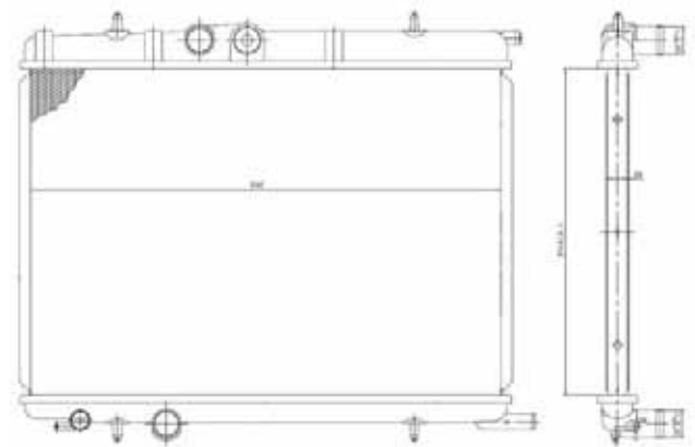
TYC 726-0006
