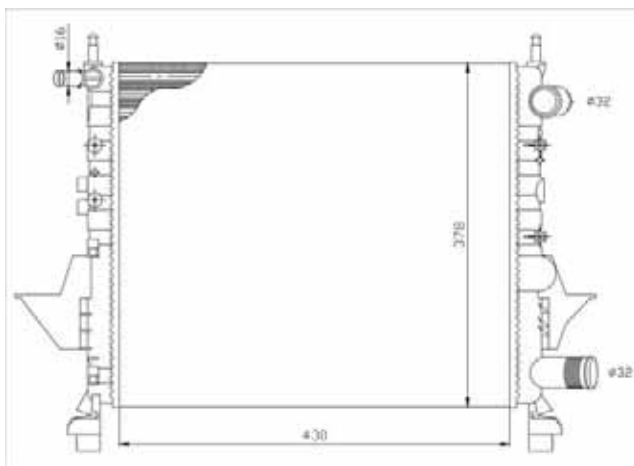
TYC 728-0041
