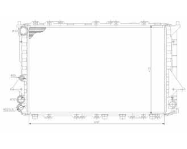
TYC 702-0027
