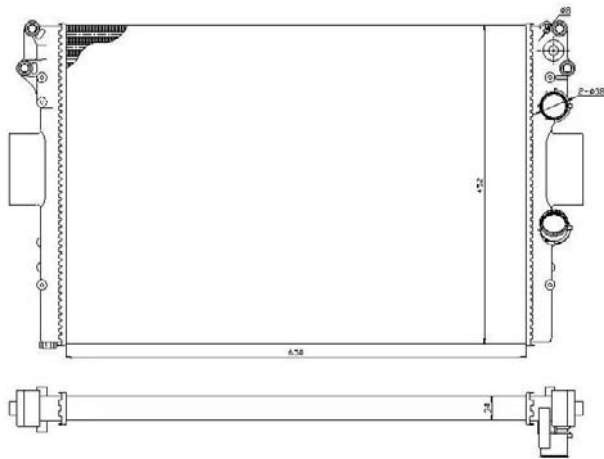
TYC 715-0001-R
