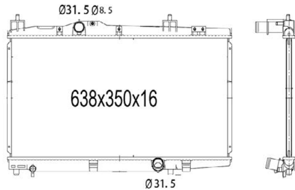
TYC 736-1008
