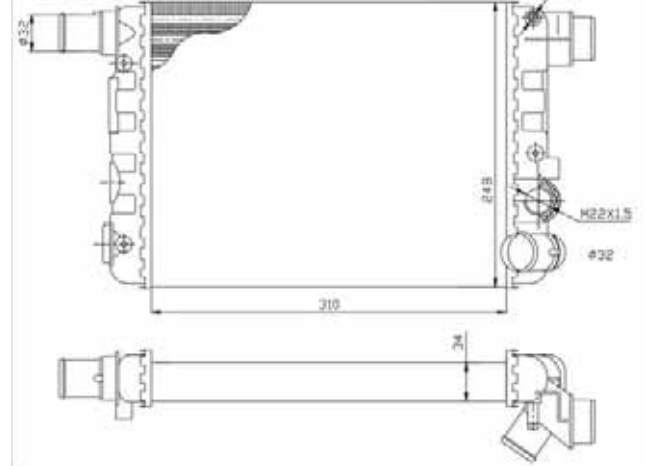
TYC 709-0009
