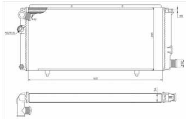
TYC 726-0014-R
