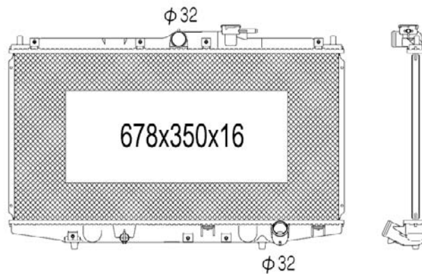
TYC 712-1002
