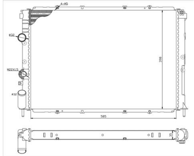
TYC 728-0025-R
