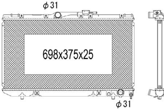
TYC 736-1027
