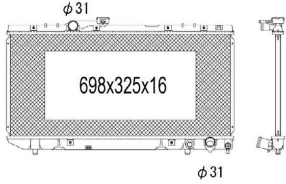
TYC 736-1004
