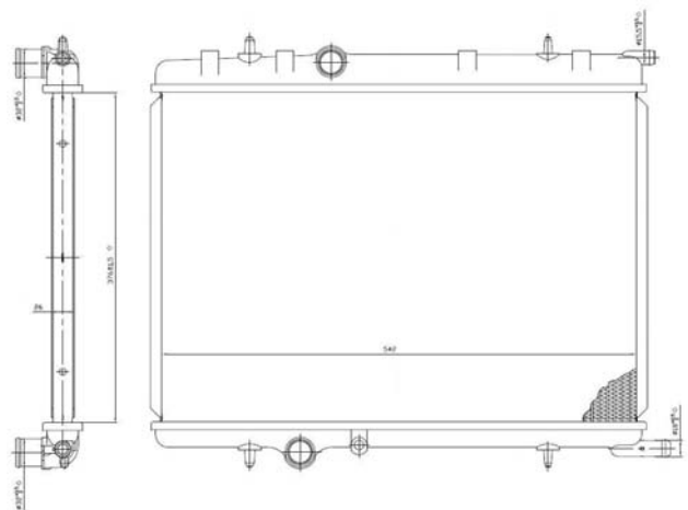
TYC 705-0027
