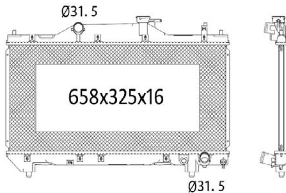
TYC 736-1018
