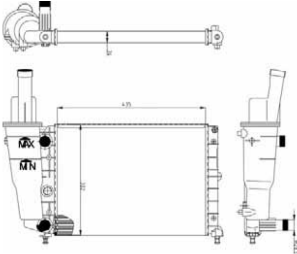
TYC 709-0004
