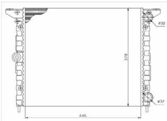
TYC 737-0015
