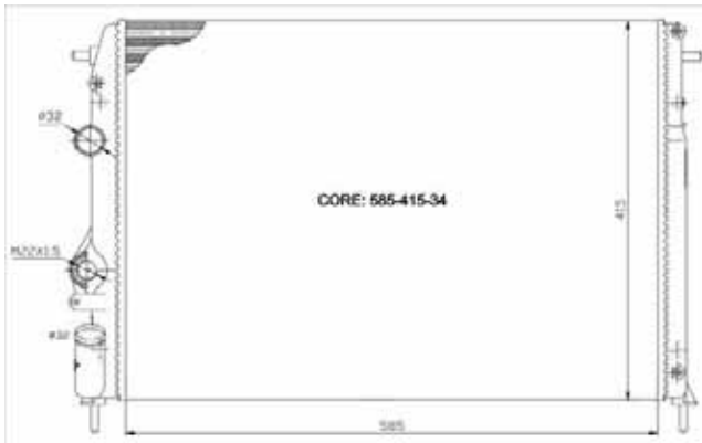
TYC 728-0011
