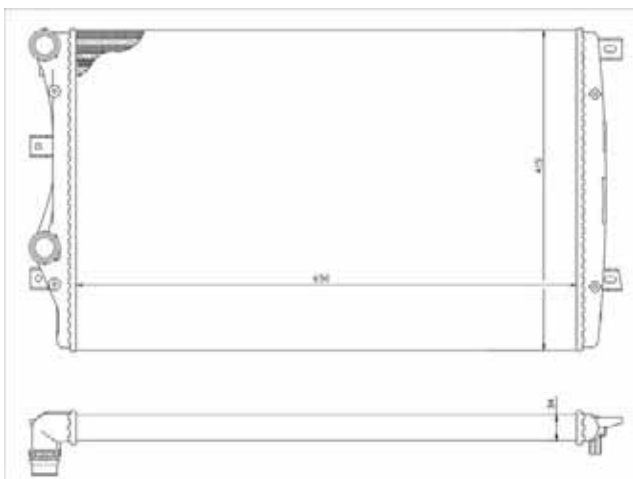
TYC 737-0017-R
