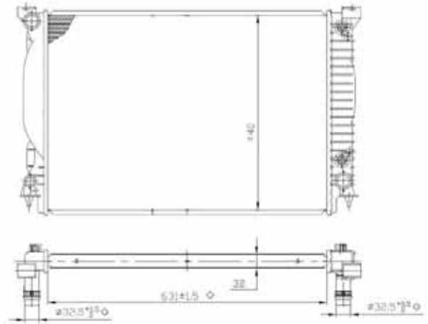
TYC 702-0021
