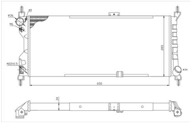
TYC 725-0019-R
