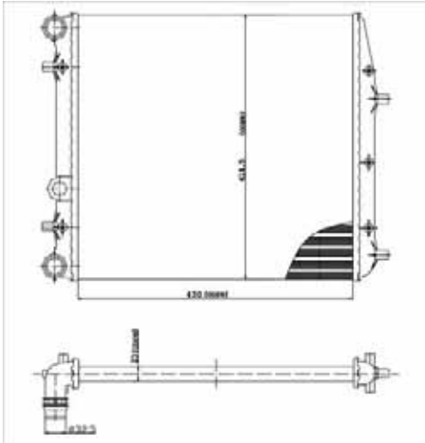
TYC 737-0013
