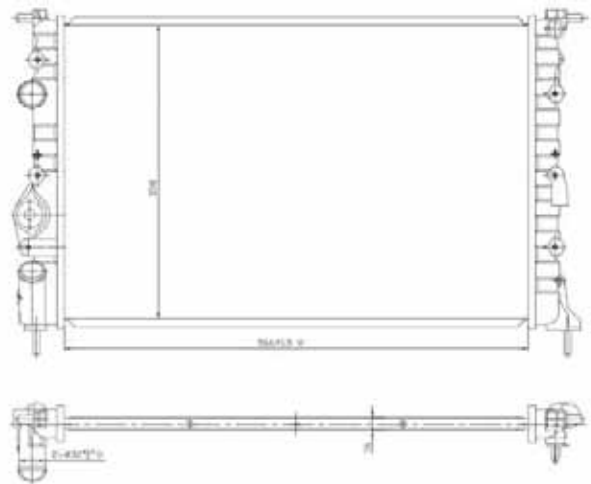
TYC 728-0027
