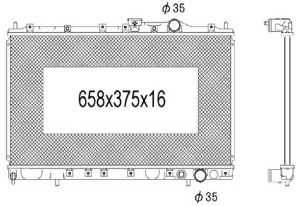
TYC 723-1001
