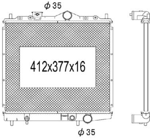
TYC 723-1015
