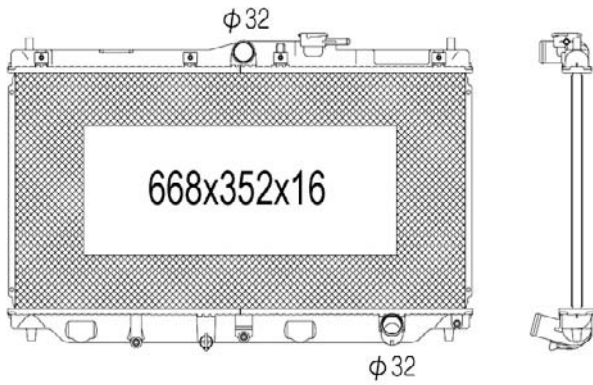
TYC 712-1007
