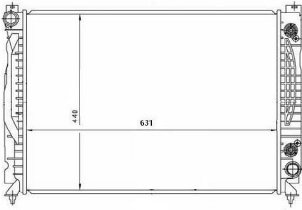
TYC 702-0001
