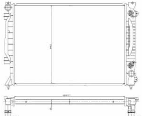
TYC 702-0018
