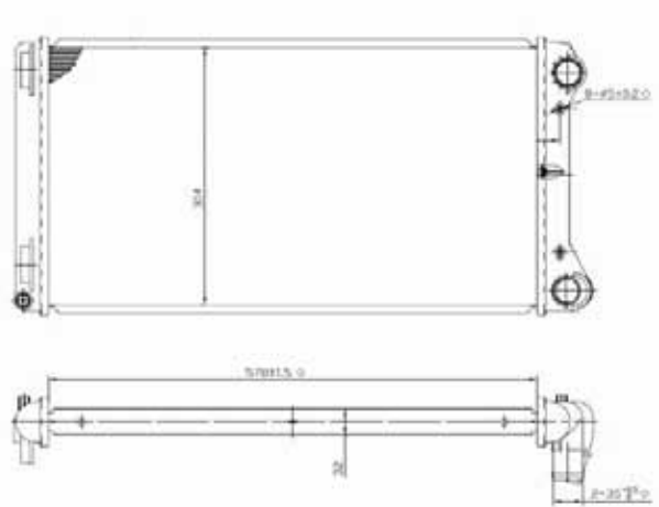
TYC 709-0002
