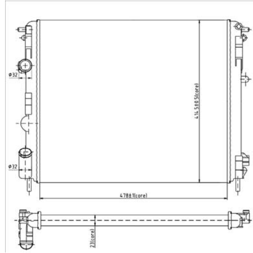
TYC 728-0010
