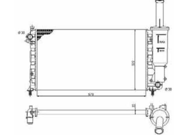
TYC 709-0013
