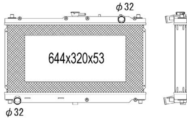
TYC 720-1005
