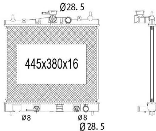
TYC 724-1014
