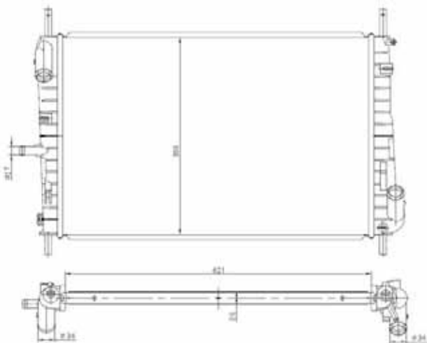
TYC 710-0047
