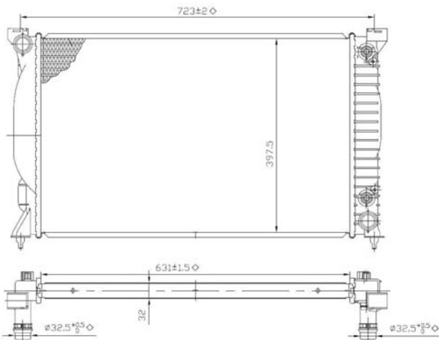
TYC 702-0022
