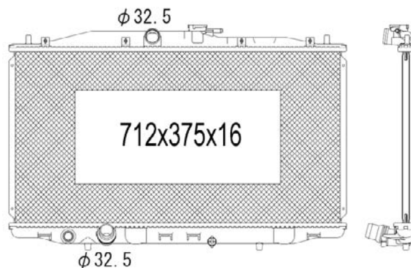
TYC 712-1004
