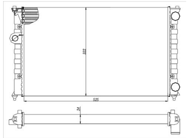
TYC 737-0016
