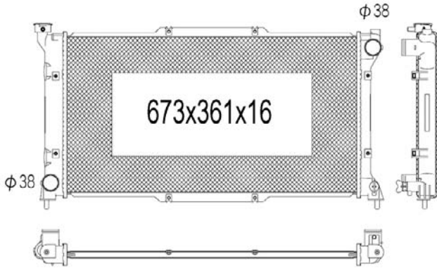
TYC 734-1003
