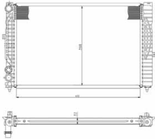
TYC 702-0034
