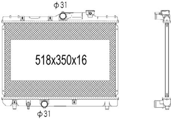
TYC 736-1005
