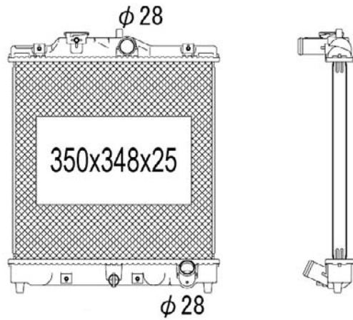
TYC 712-1008
