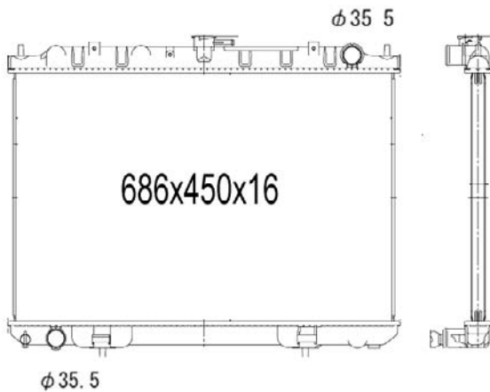
TYC 724-1013
