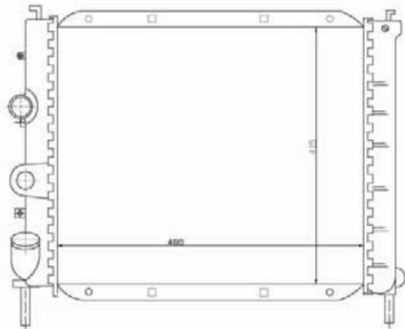
TYC 728-0008-R
