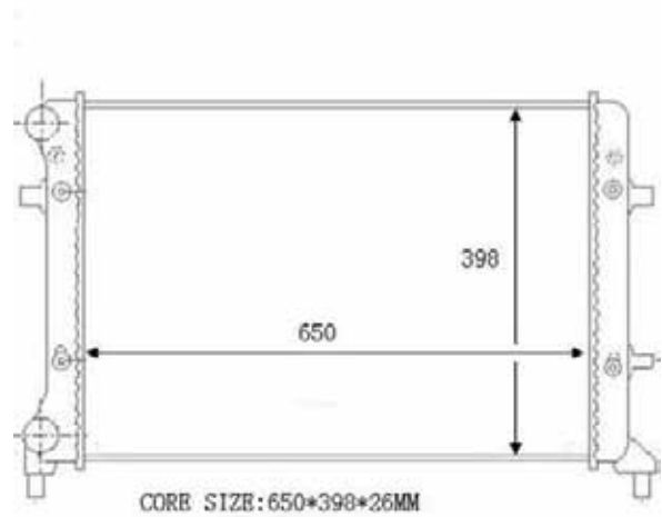
TYC 702-0023
